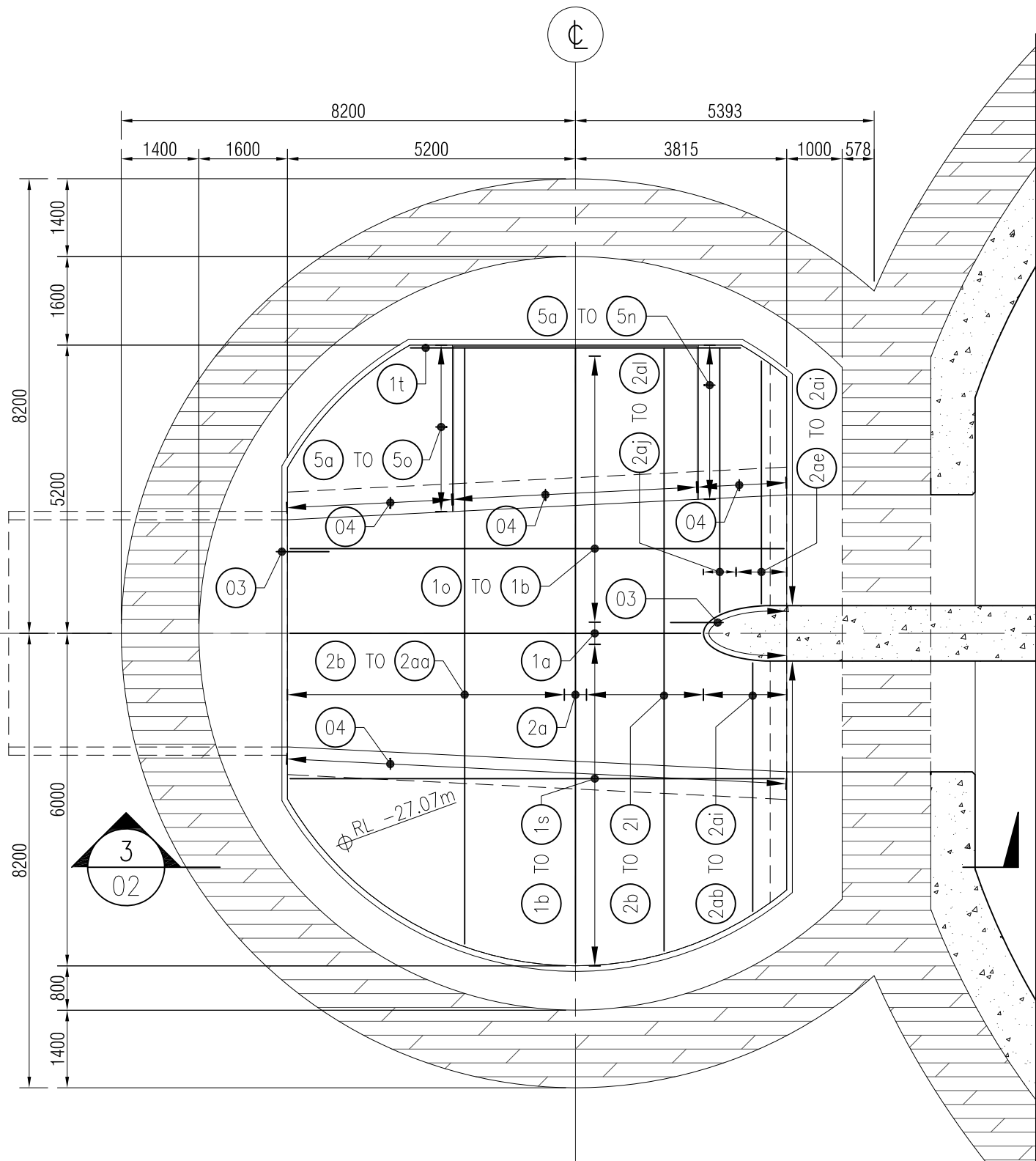
BASE SLAB TOP & BOTTOM LAYER LAYOUT @ RL -27.07m SCALE: 1:100
