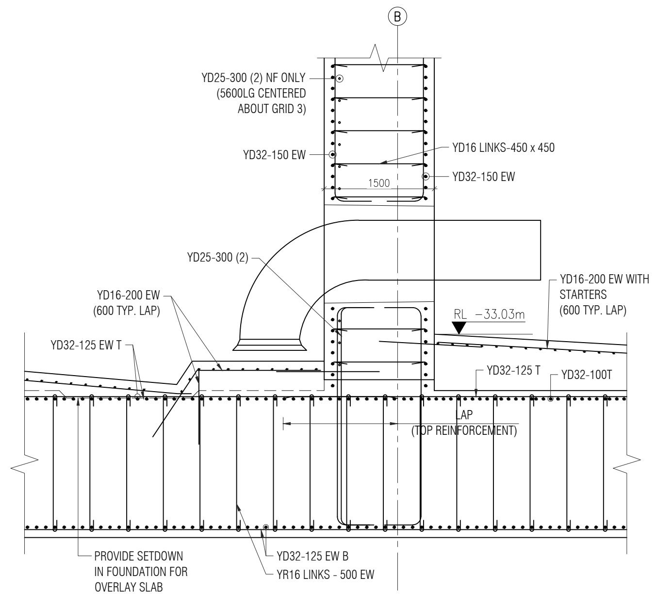
SECTION 14 SCALE: 1:50 ST-03
