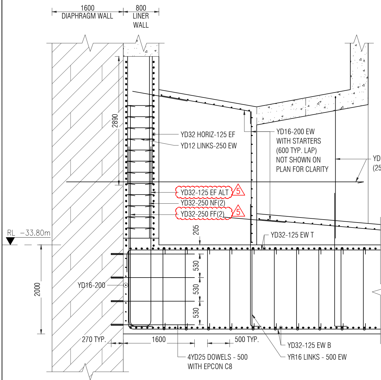
SECTION 8 SCALE: 1:50 ST-03
