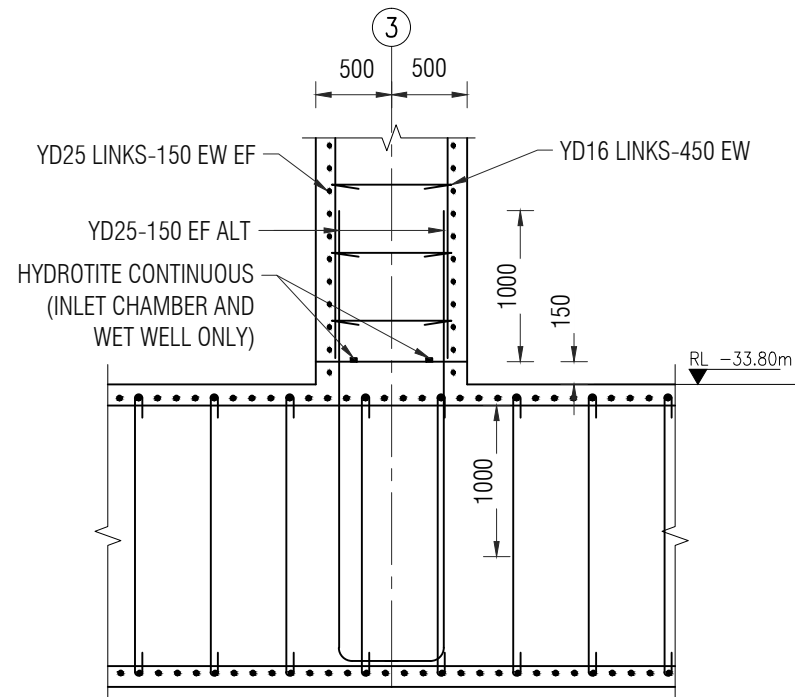
SECTION 12 SCALE: 1:50 ST-03
