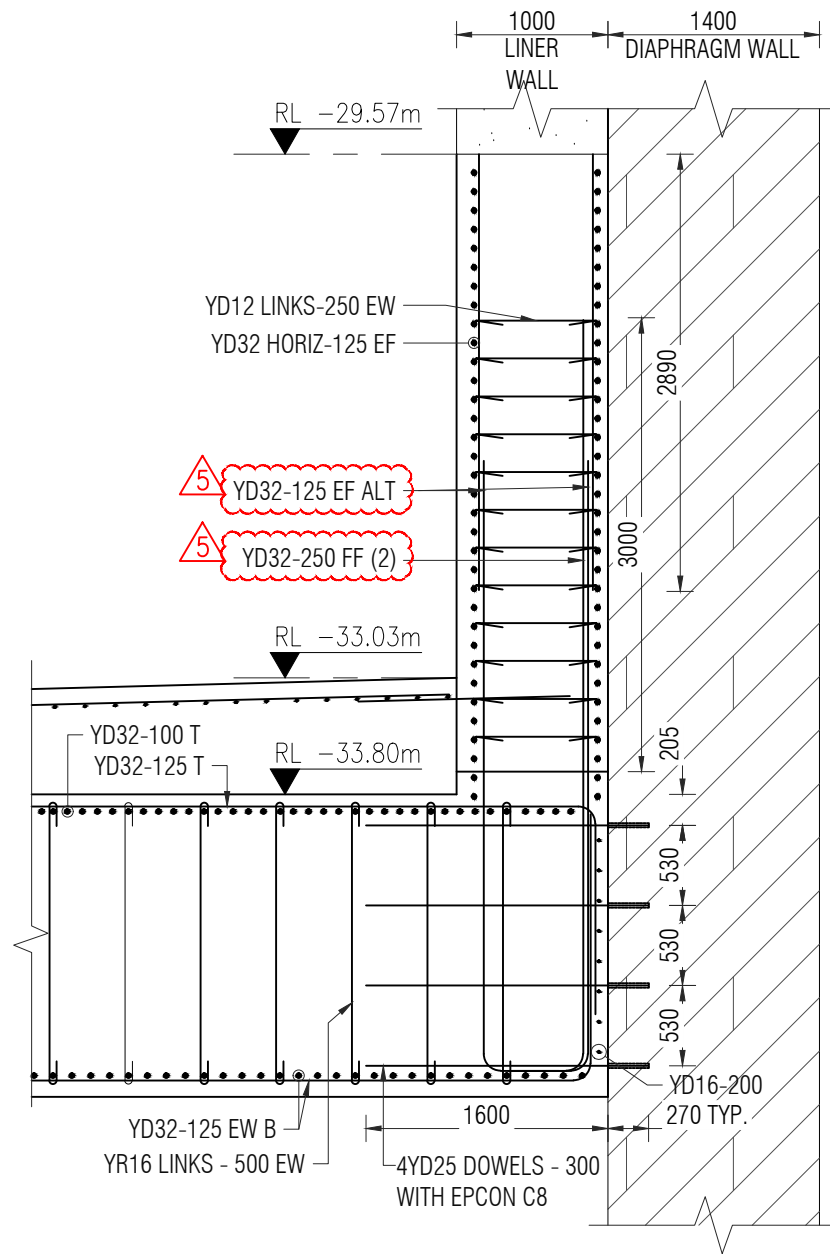
SECTION 10 SCALE: 1:50 ST-03
