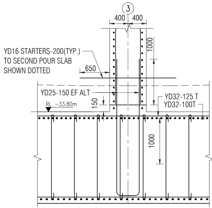
SECTION 13 SCALE: 1:50 ST-03
