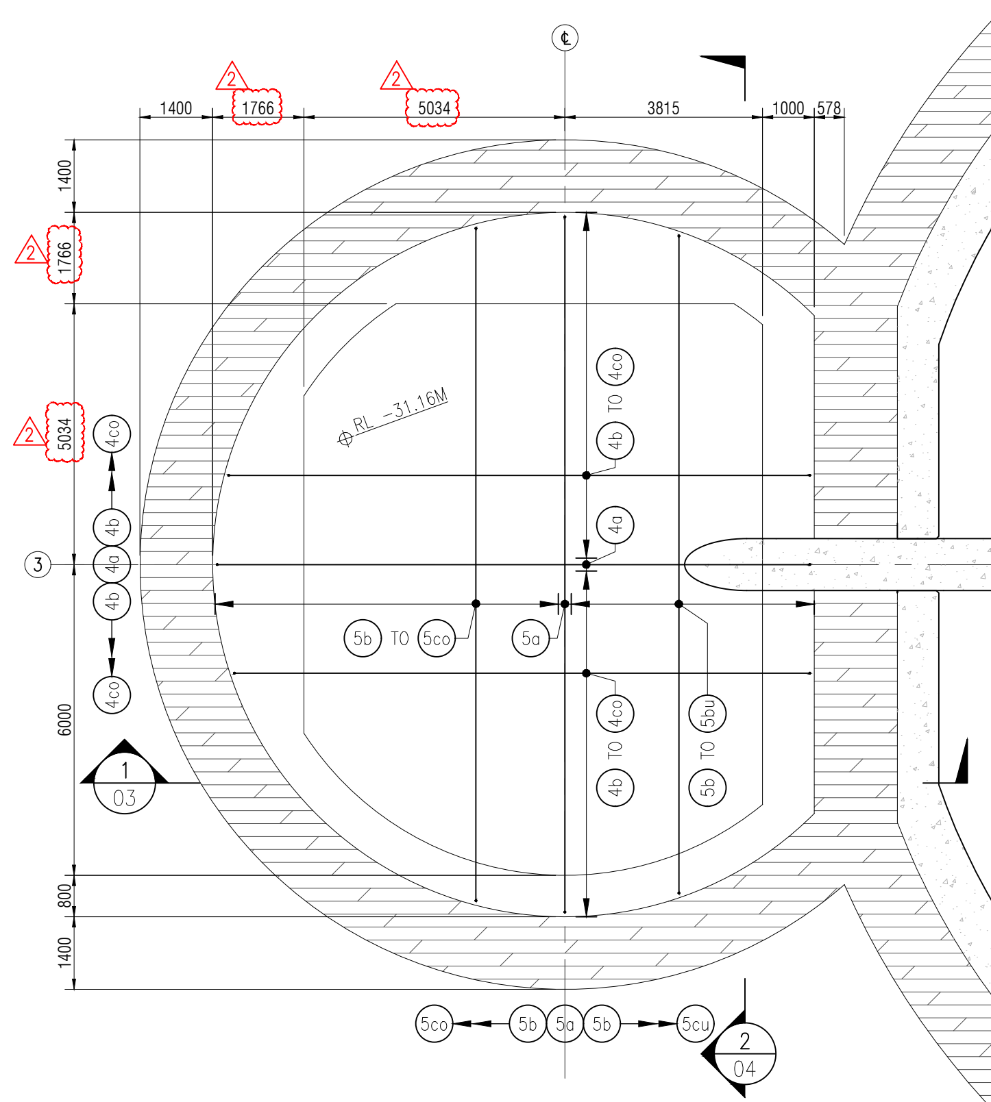
BASE SLAB TOP LAYER (T1&T2) LAYOUT @ RL - 31.16M SCALE: 1:100
