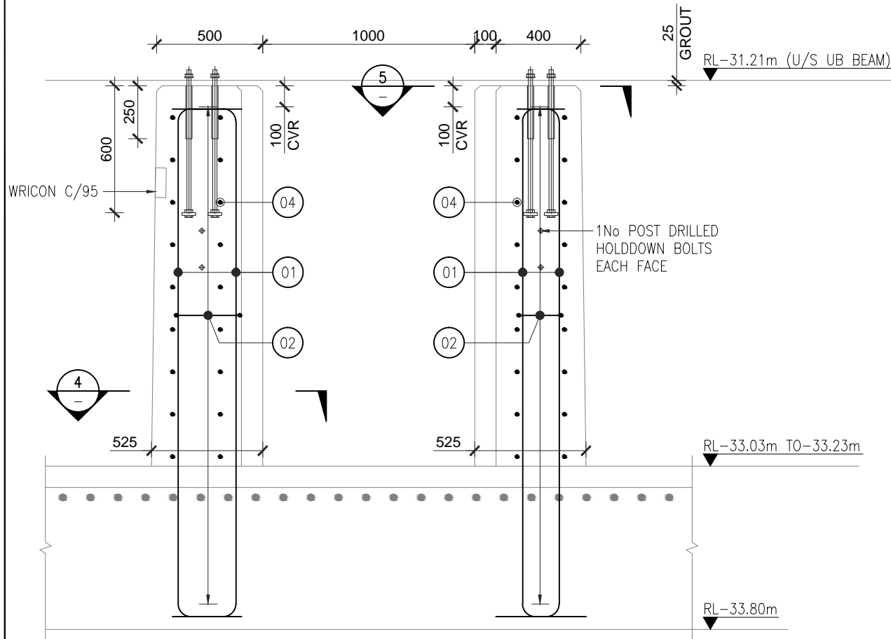
ELEVATION 3 PIPE SUPPORT CP3 (12No) SCALE: 1:25
