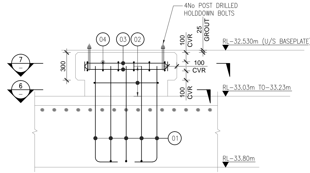
ELEVATION 4 PIPE SUPPORT CP4 (6No) SCALE: 1:25
