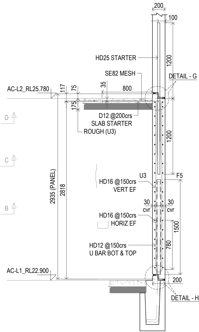
SECTION A-A SCALE 1:30
